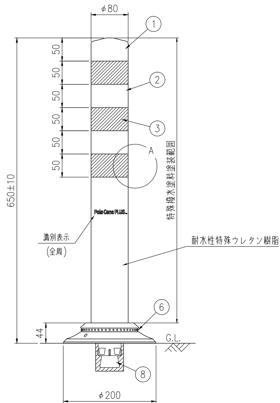
設置図 S=1/5
