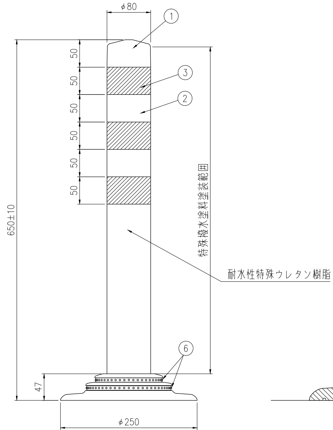
姿図 S=1/4
