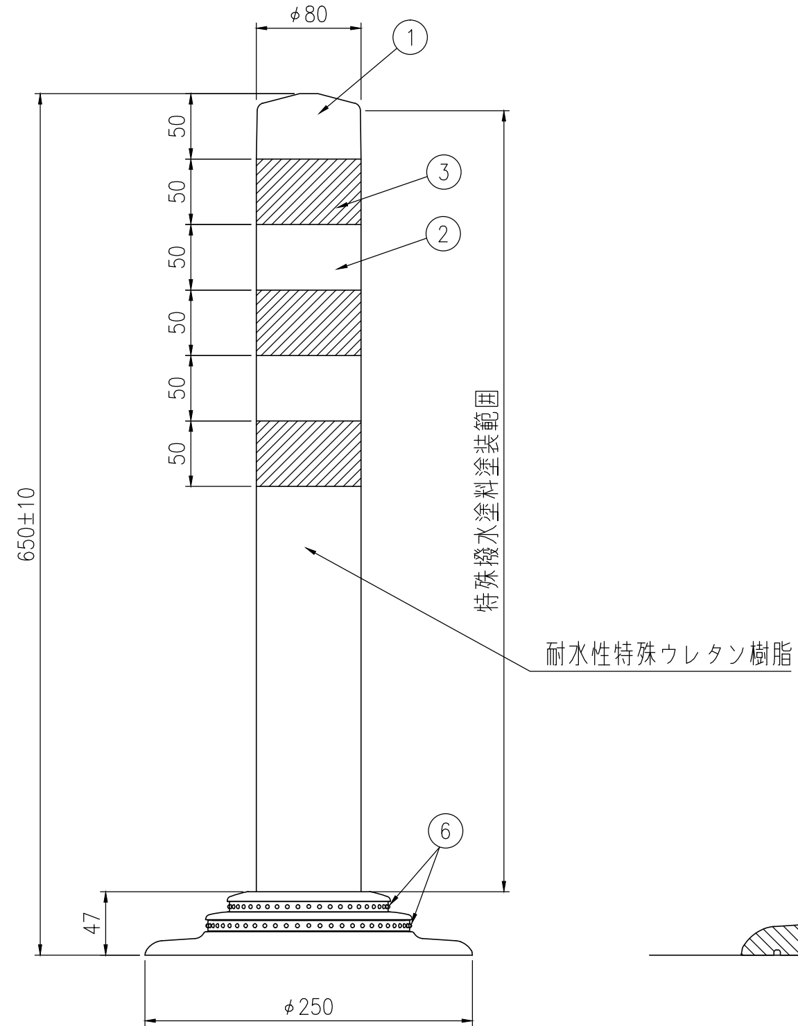
姿図 S=1/4
