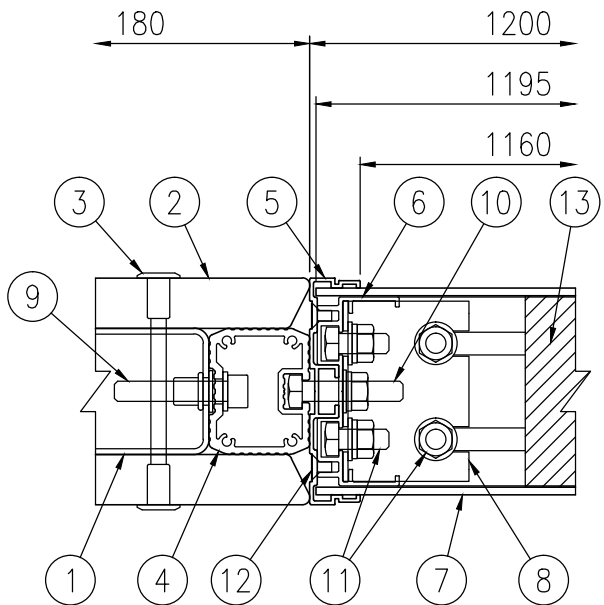
断面詳細 S=1/3
