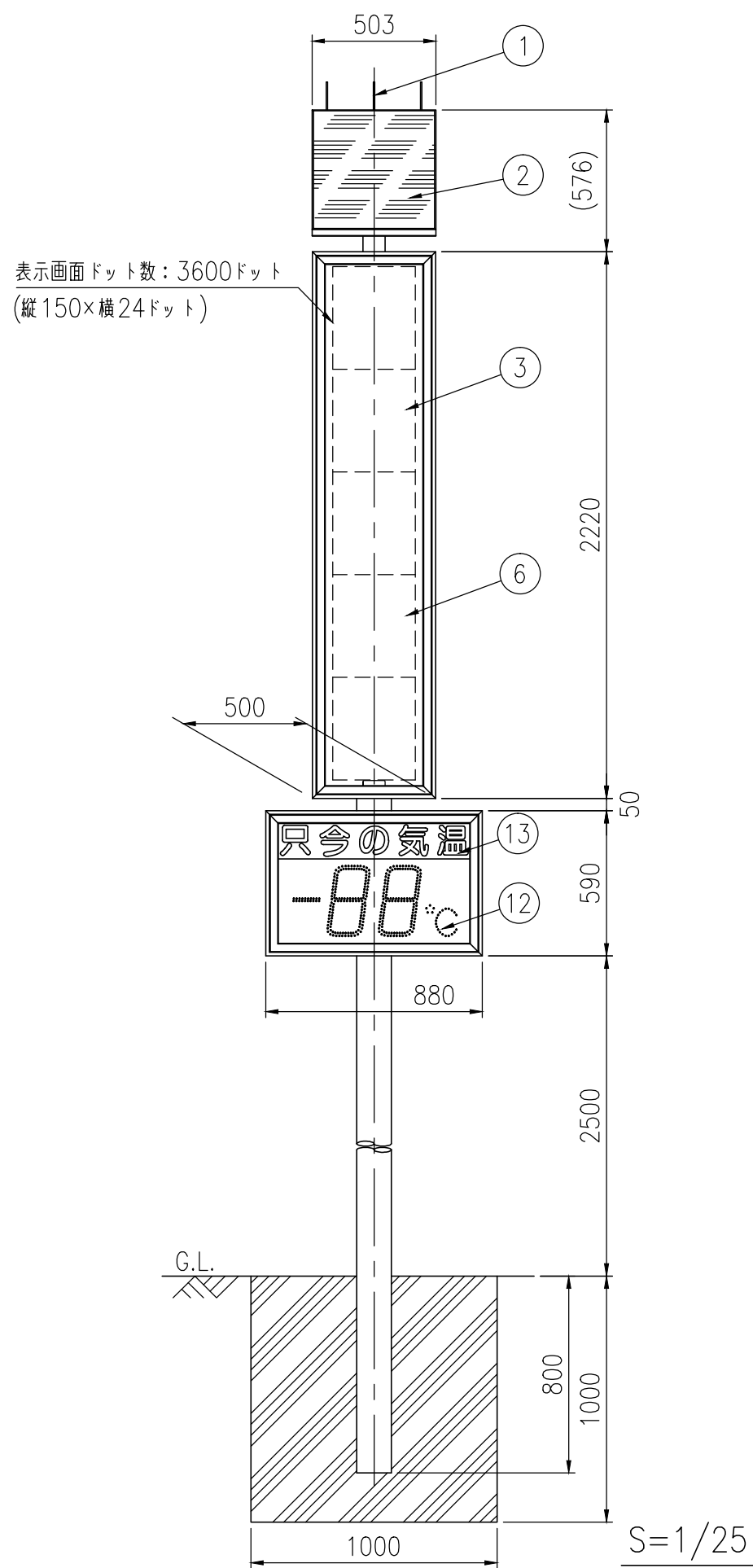
正面図
