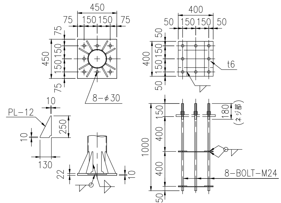
柱脚部詳細図 S=1/25
