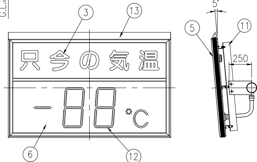
発光部 S=1/25
