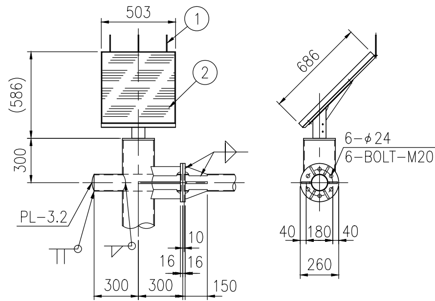
太陽電池部 S=1/25
