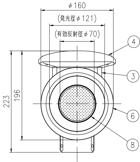
正面図
