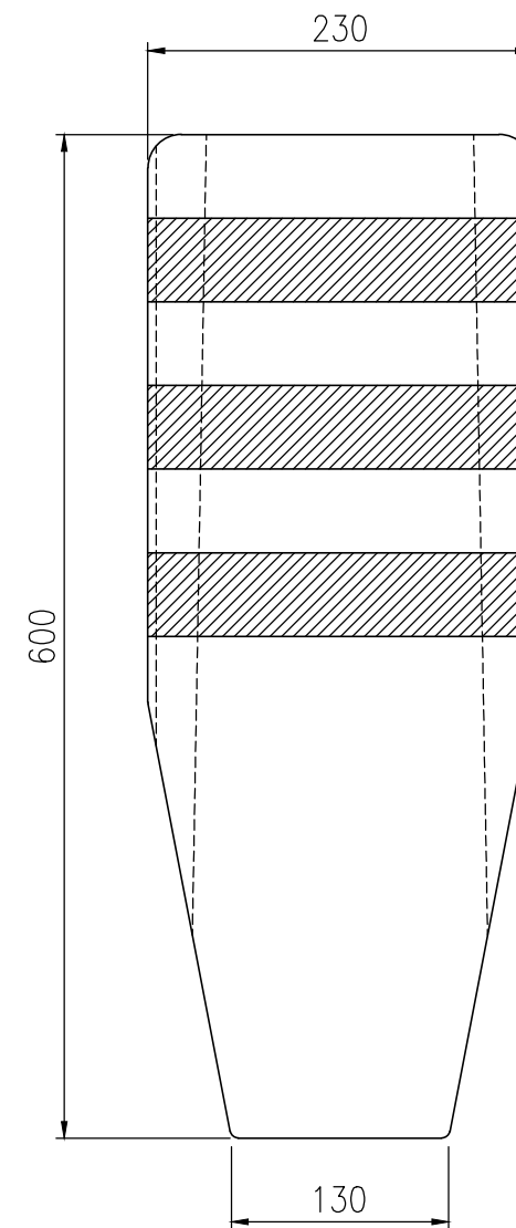
製品図 S=1/5
