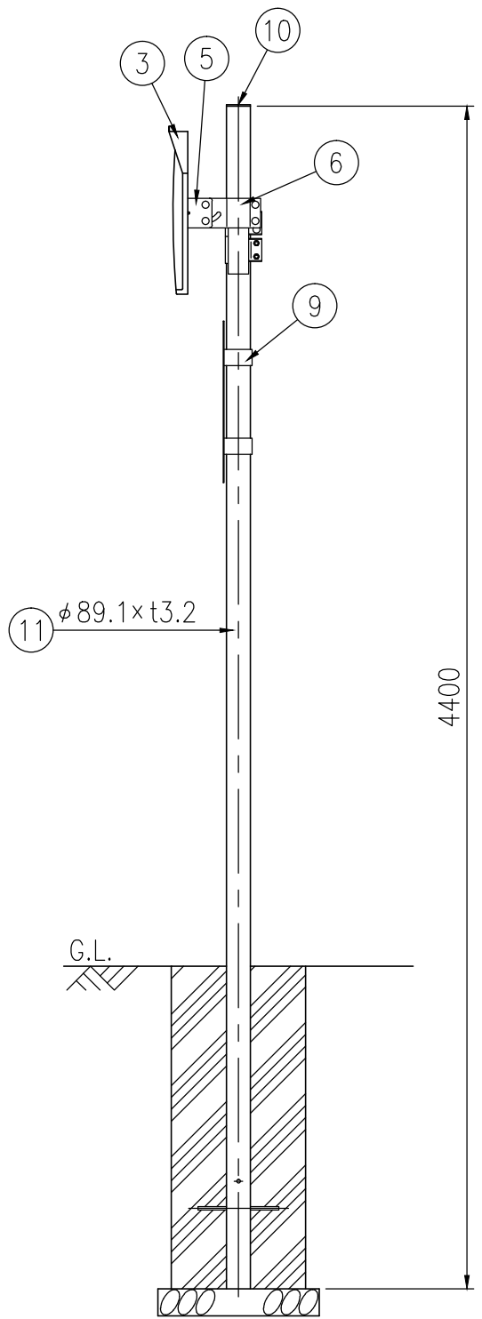
設置図 S=1/25
