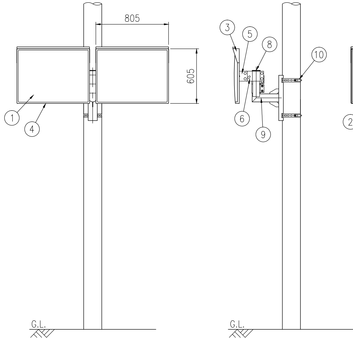
設置図 S=1/25
