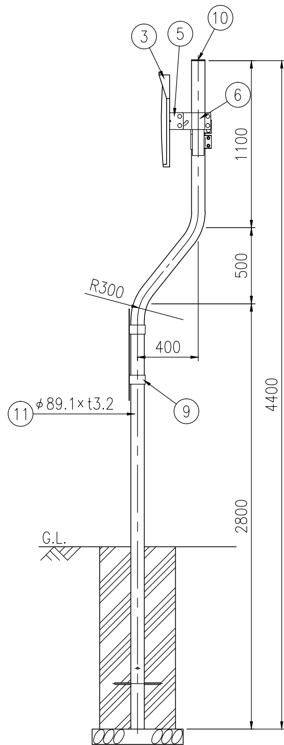
設置図 S=1/25
