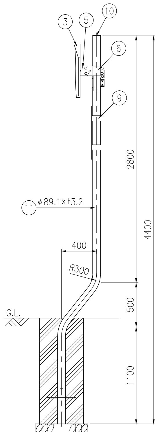
設置図 S=1/25
