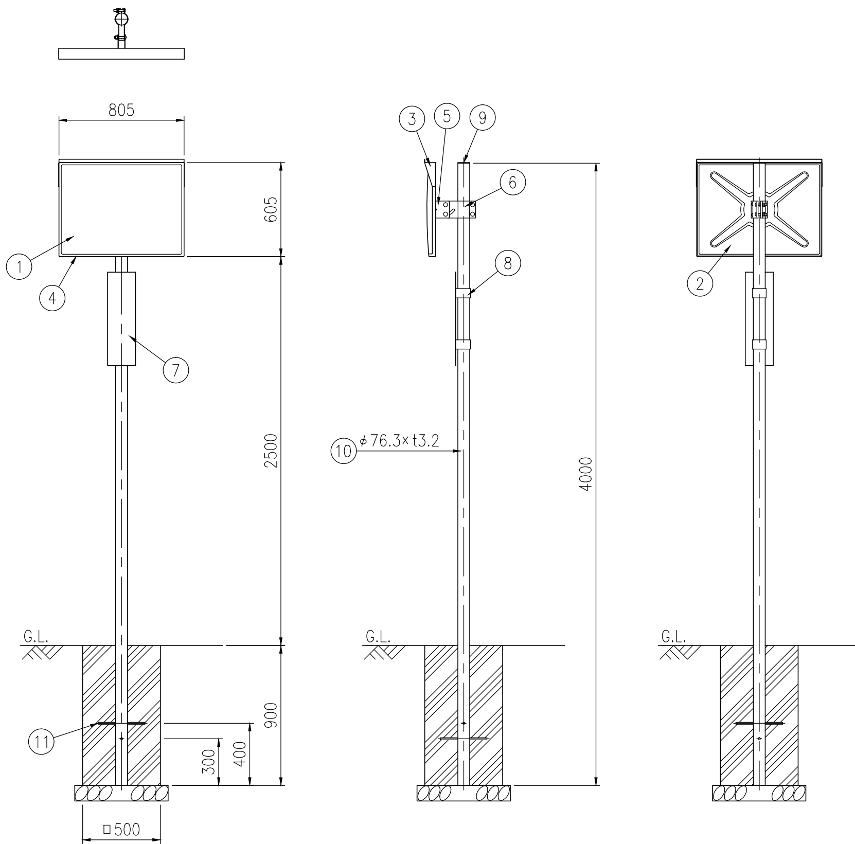
設置図 S=1/25
