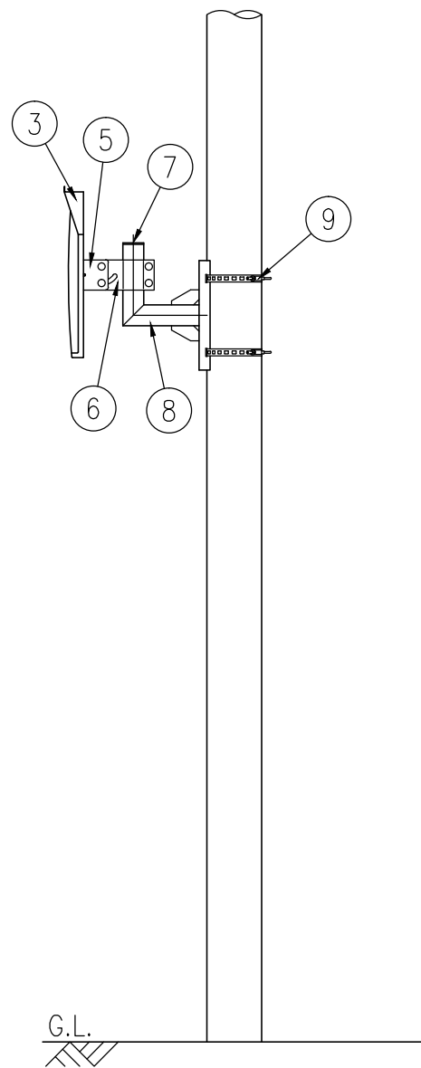
設置図 S=1/25
