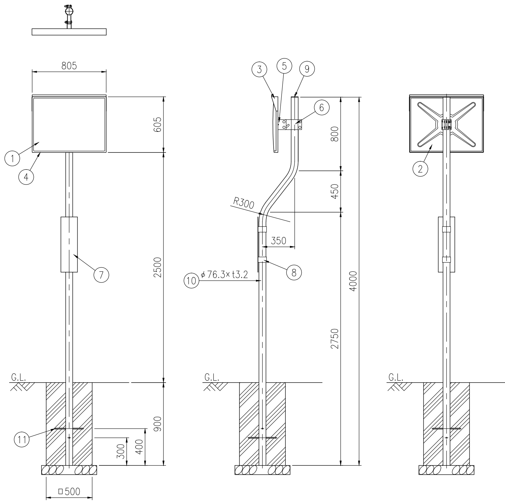
設置図 S=1/25
