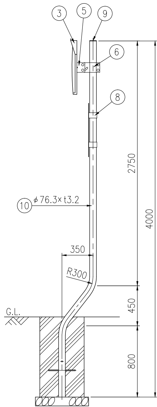
設置図 S=1/25
