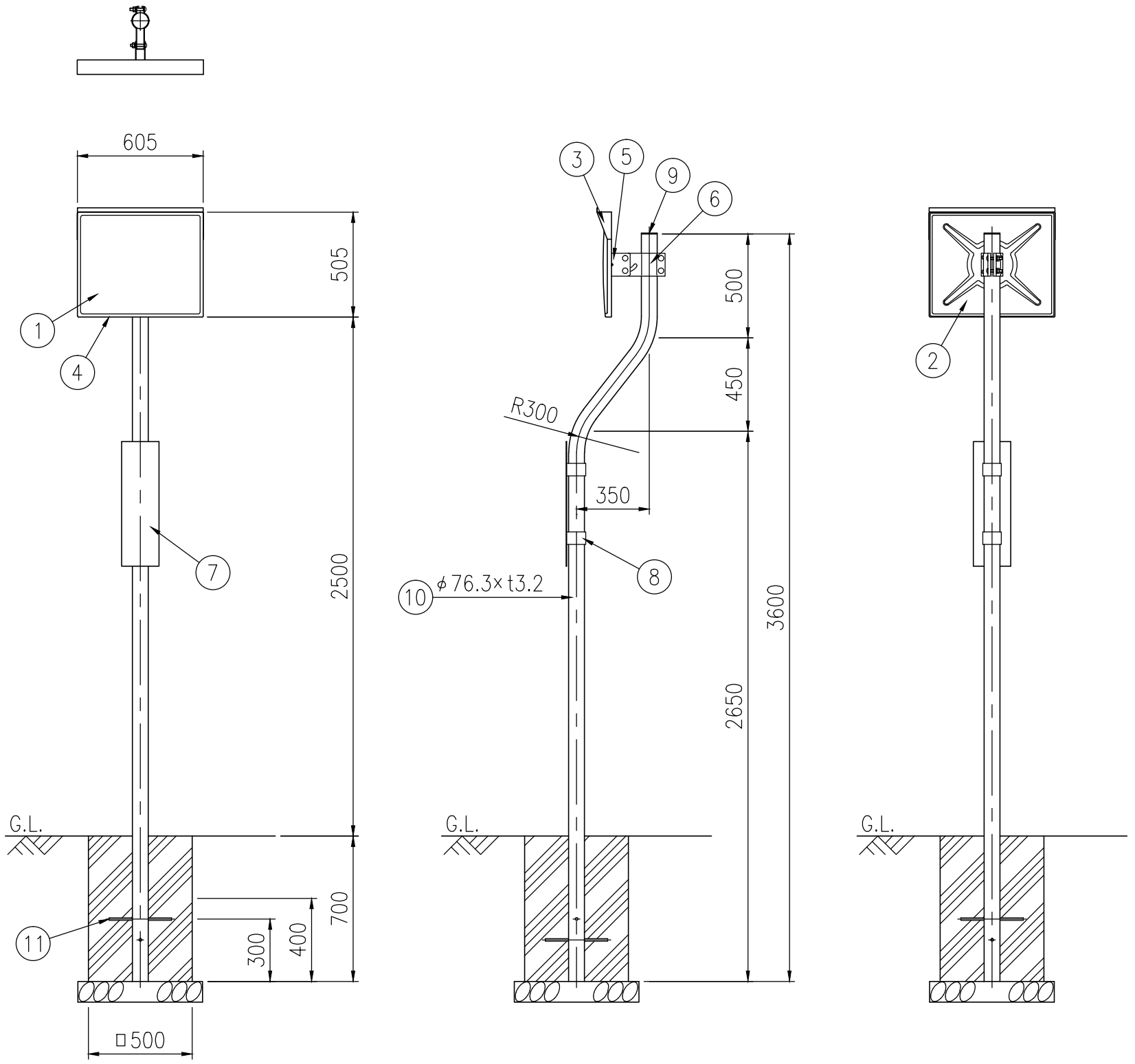
設置図 S=1/25
