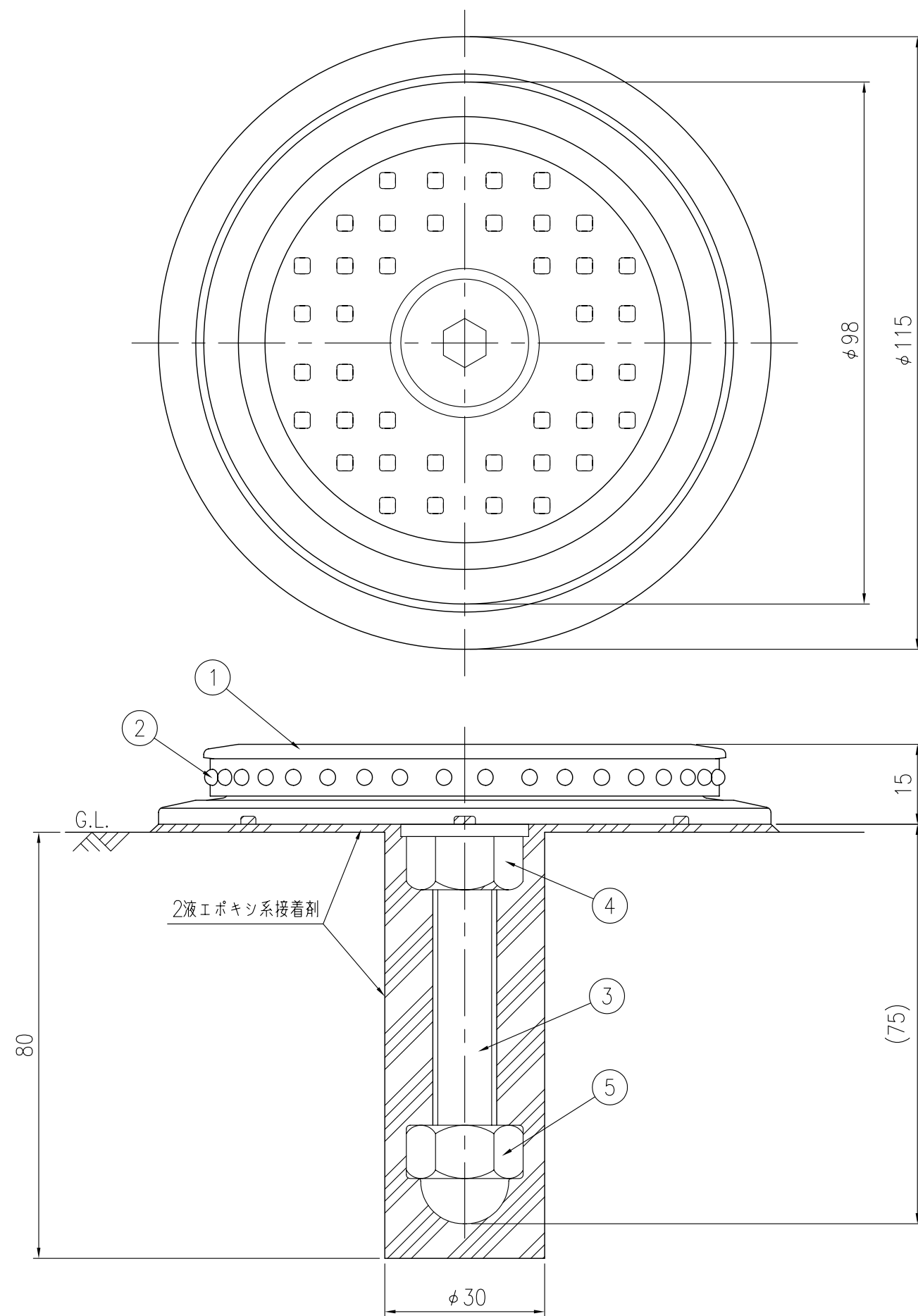
設置図 S=1/1
