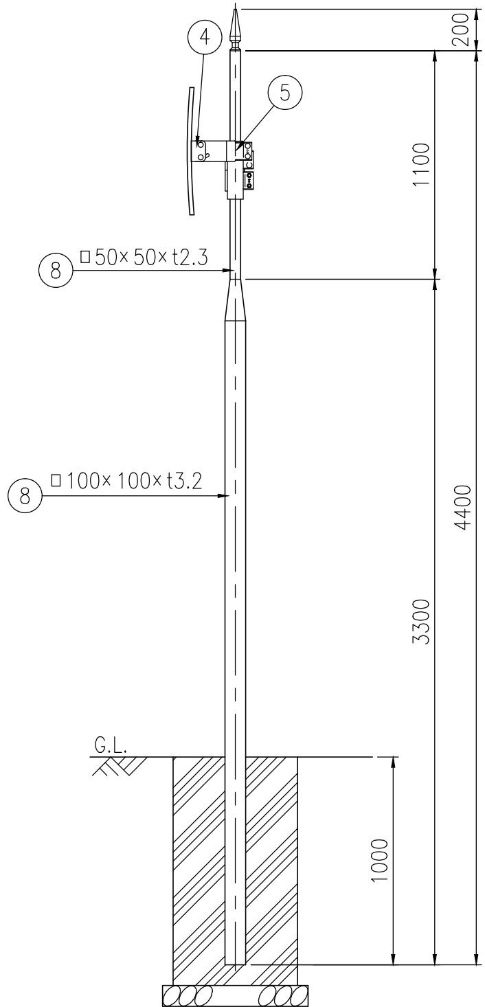
設置図 S=1/25
