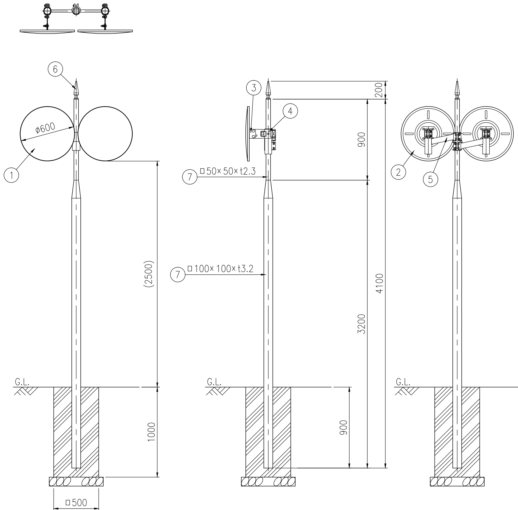
設置図 S=1/25
