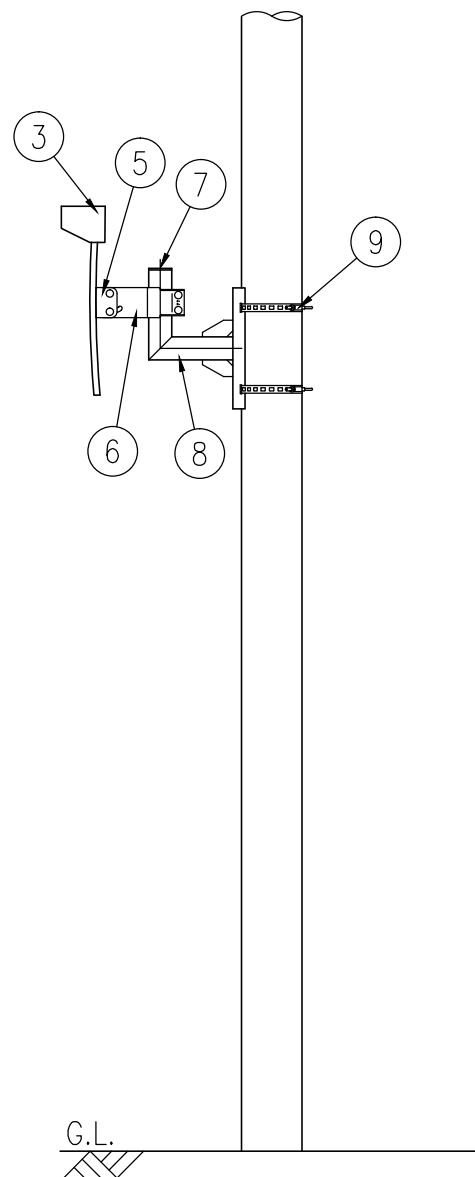
設置図 S=1/25
