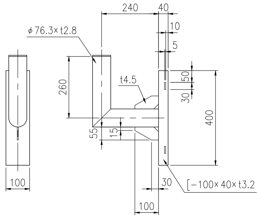
⑨ 電柱取付金具詳細図 S=1/10
