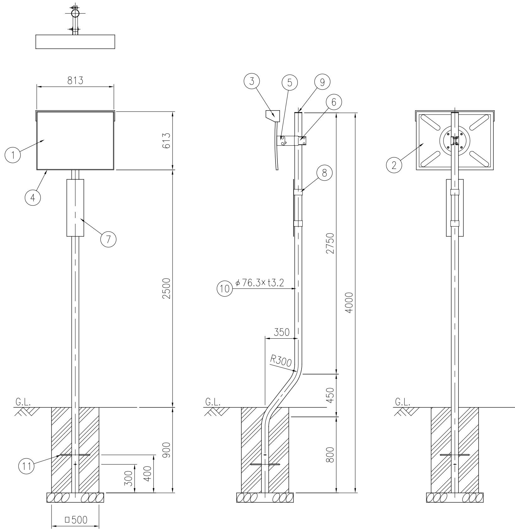
設置図 S=1/25
