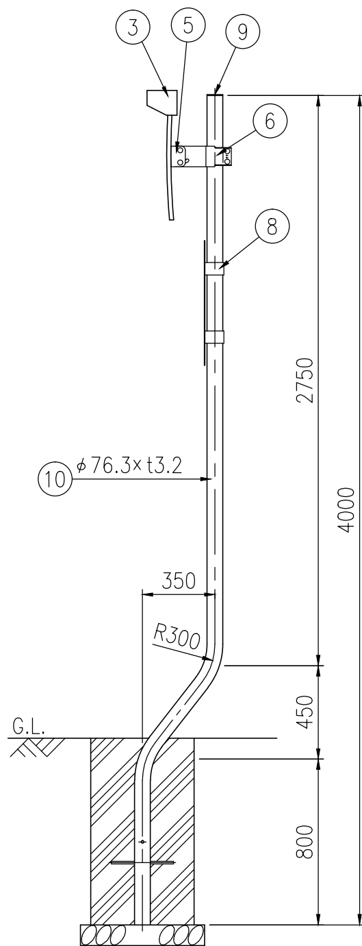
設置図 S=1/25
