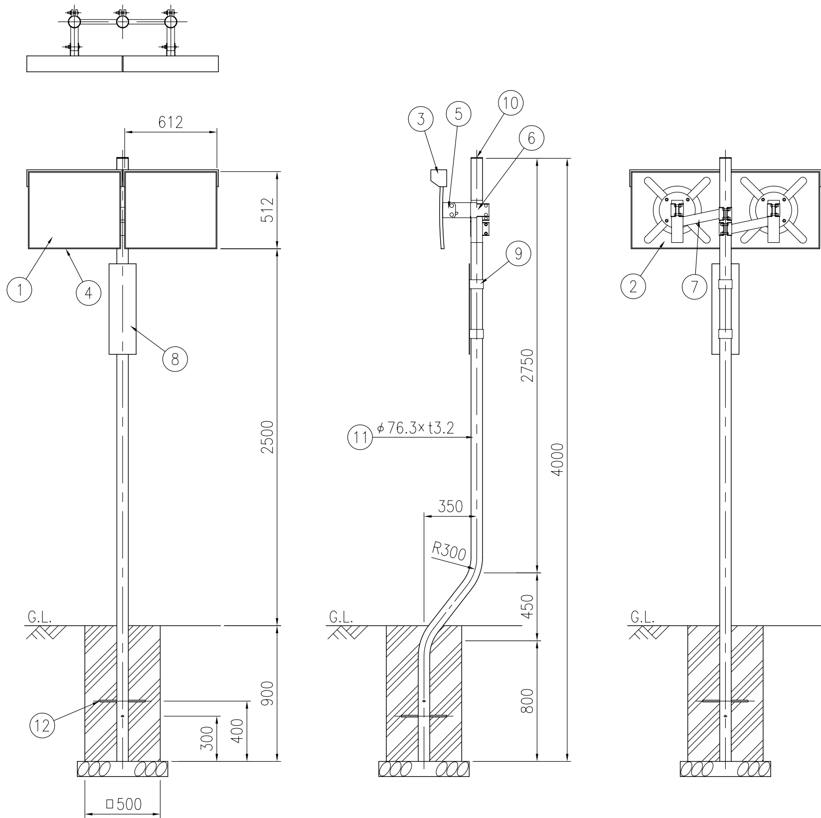
設置図 S=1/25
