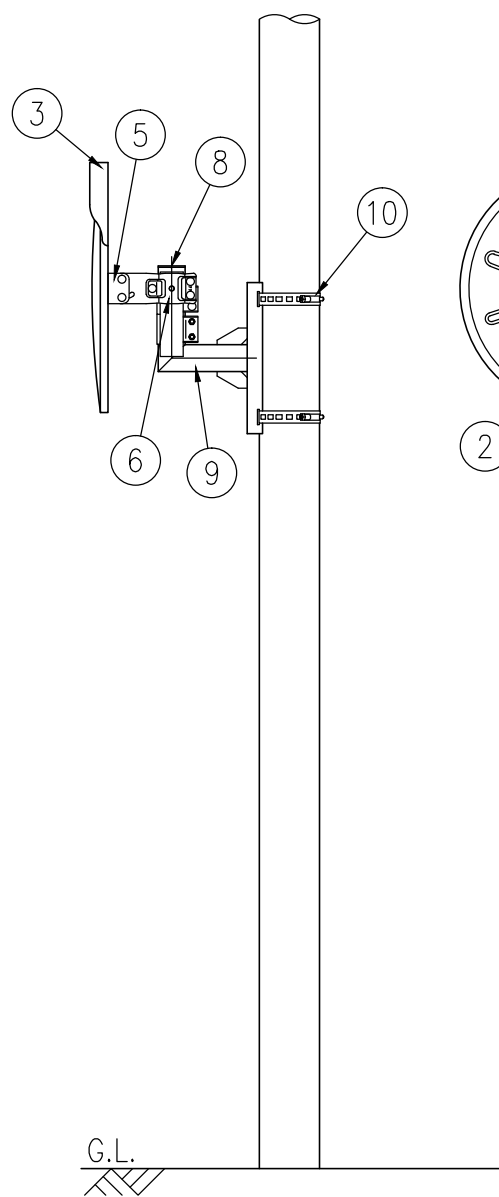
設置図 S=1/25
