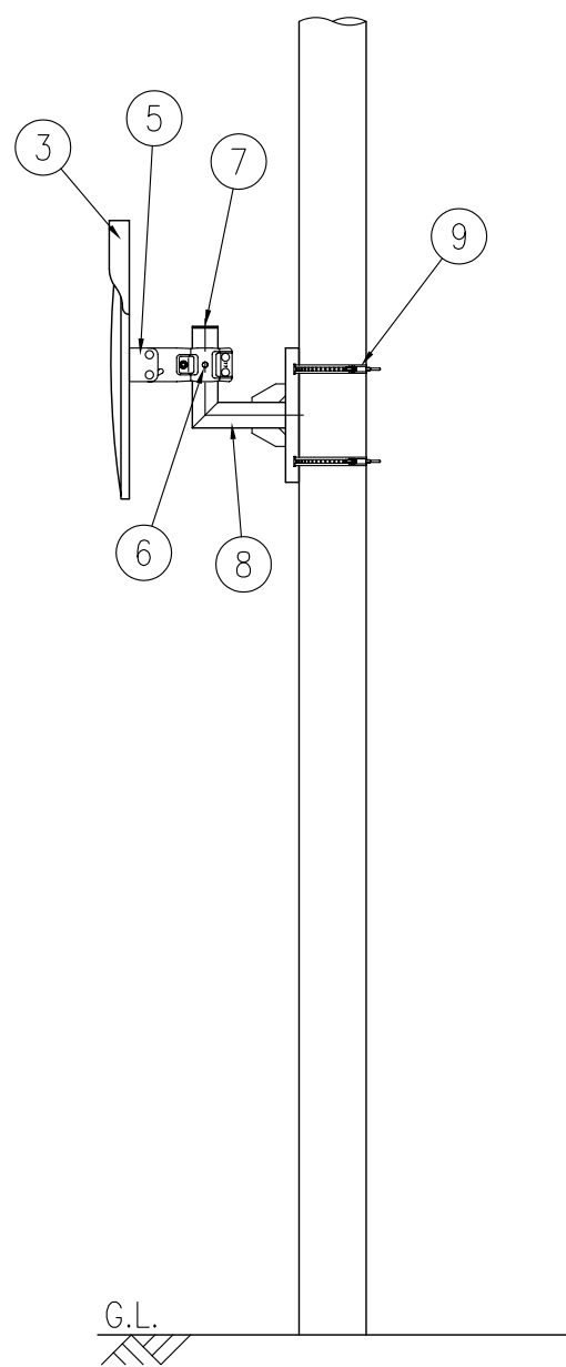
設置図 S=1/25
