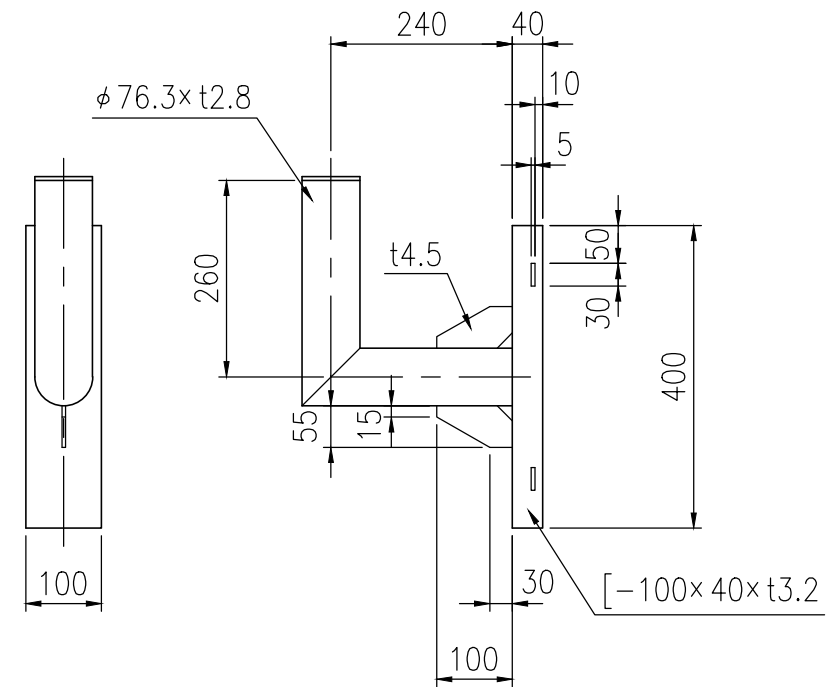
⑨ 電柱取付金具詳細図 S=1/10
