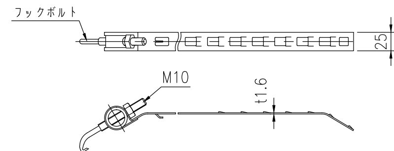
⑩ 取付バンド詳細図 S=1/5
