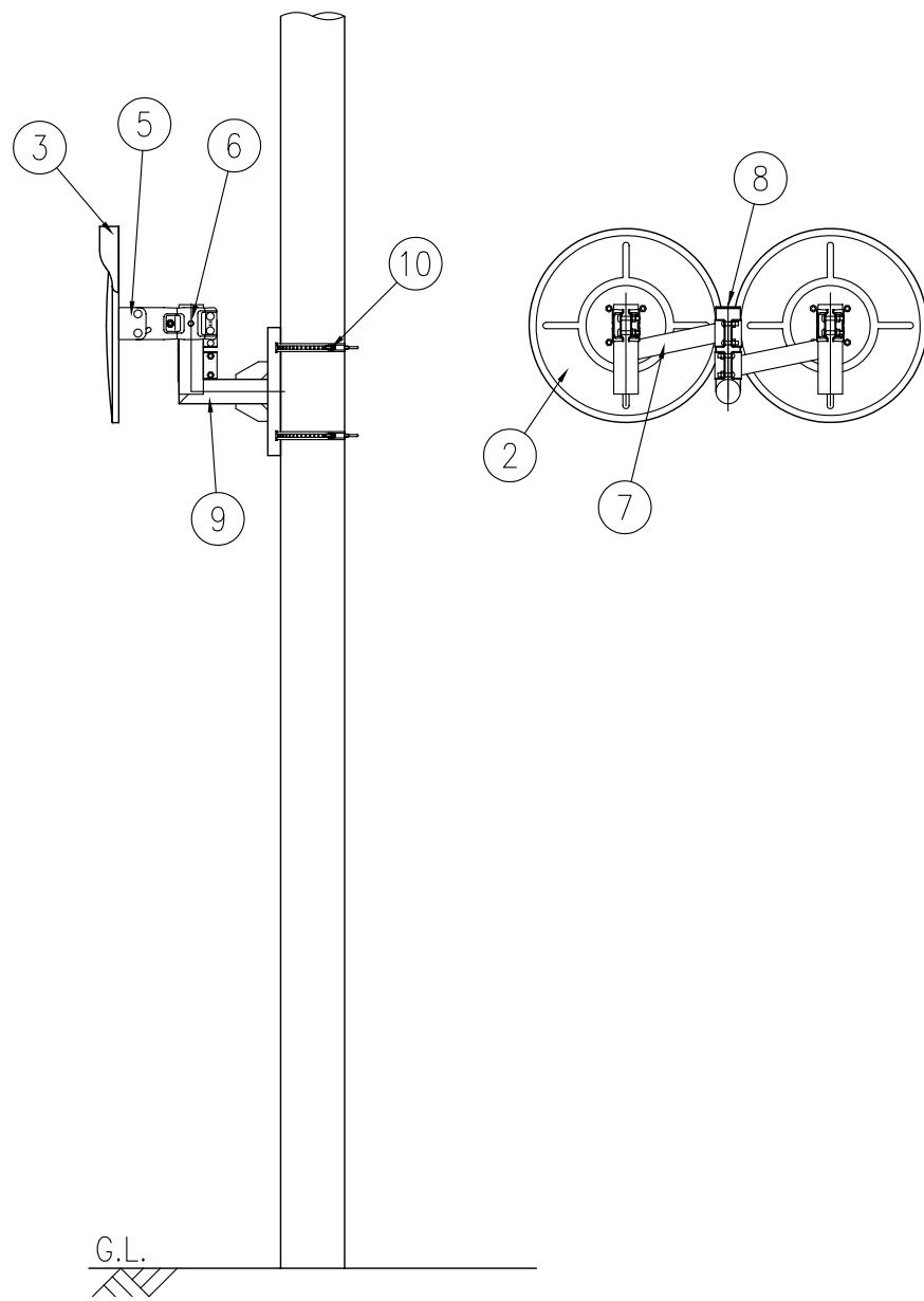
設置図 S=1/25
