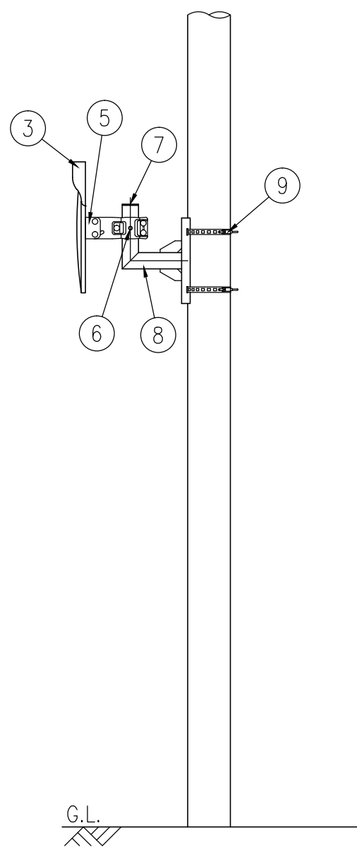
設置図 S=1/25
