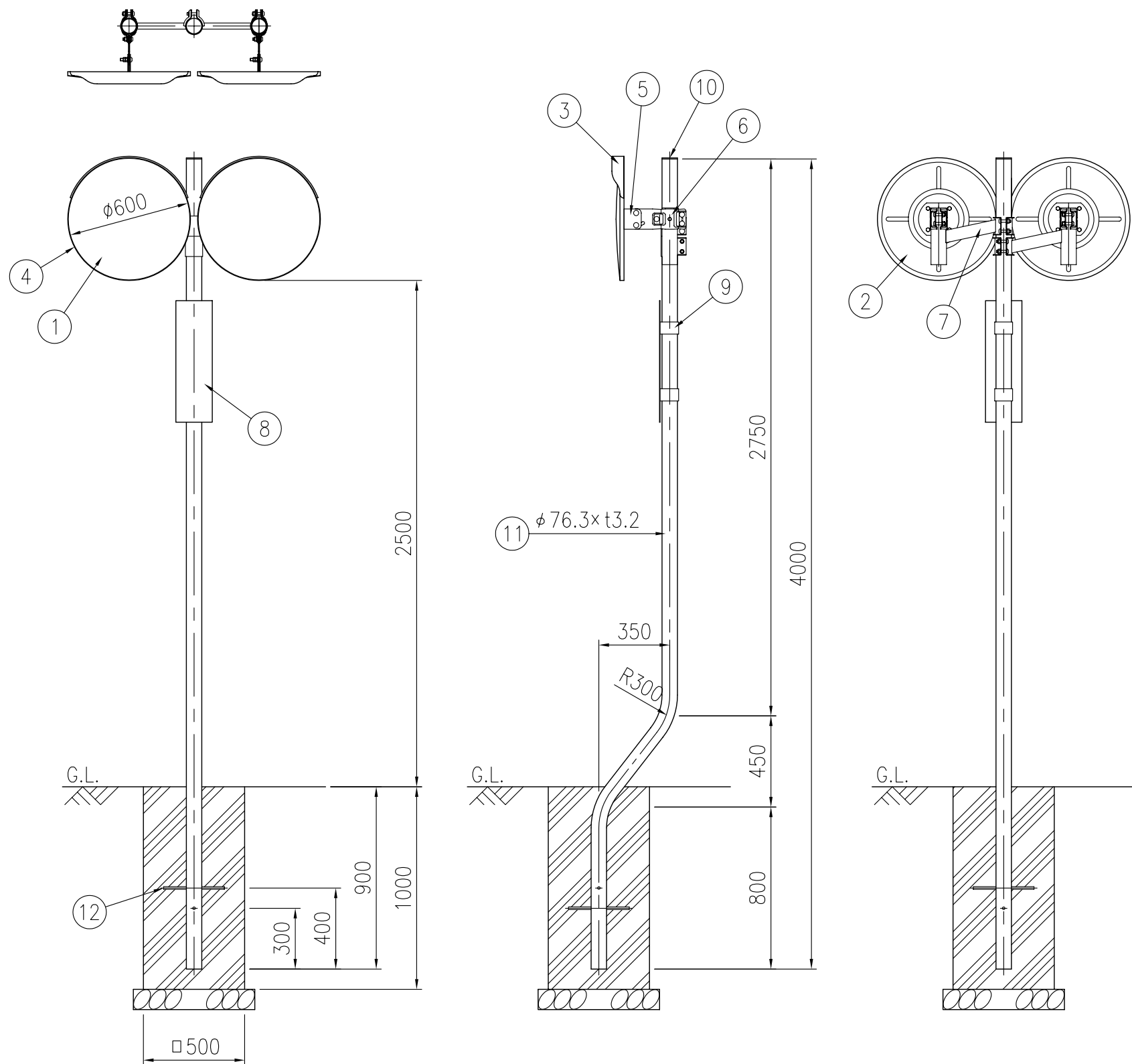
設置図 S=1/25
