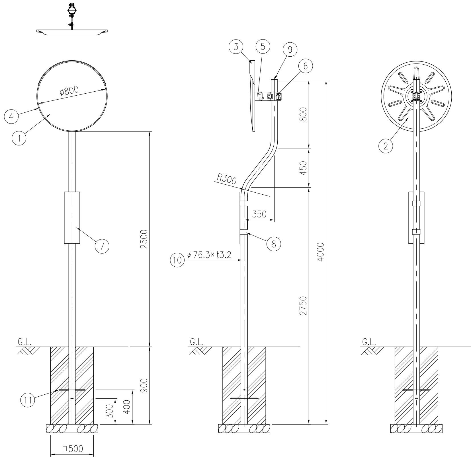
設置図 S=1/25
