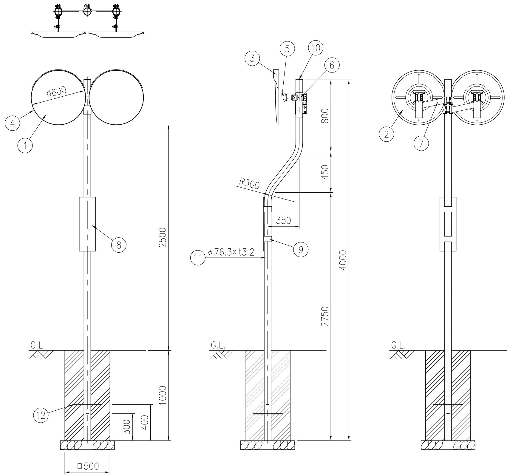
設置図 S=1/25
