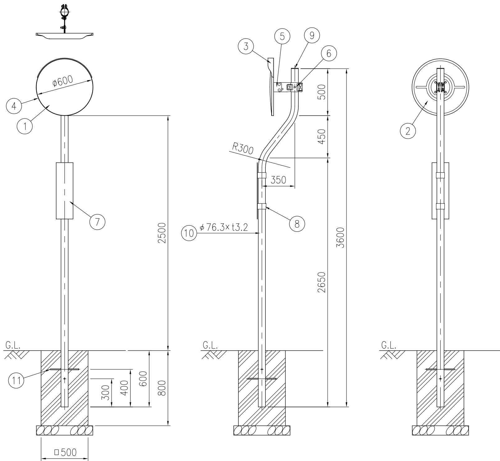
設置図 S=1/25
