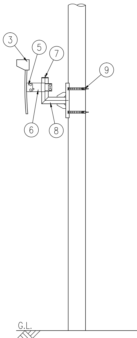
設置図 S=1/25
