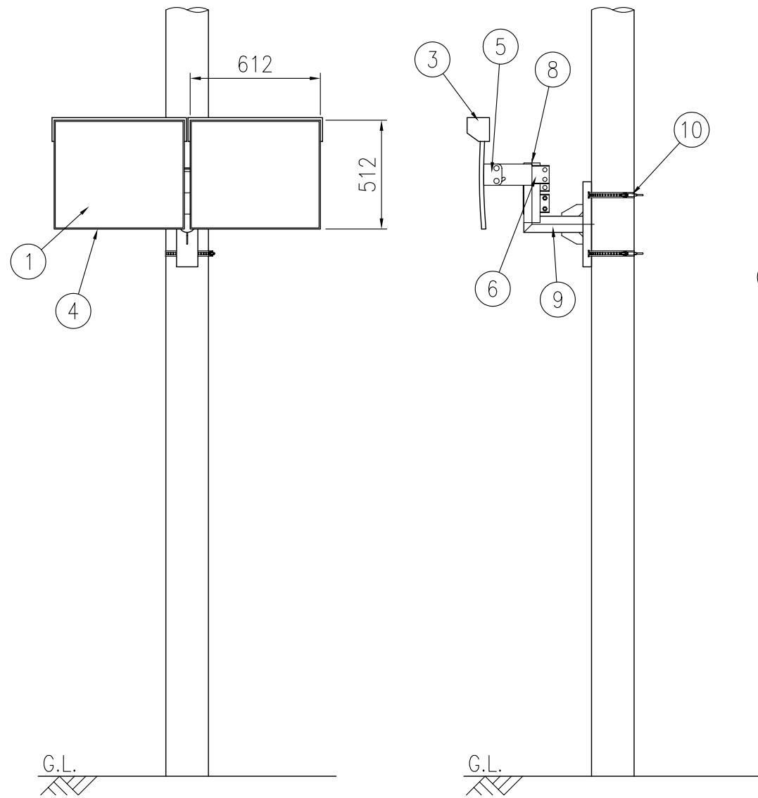
設置図 S=1/25
