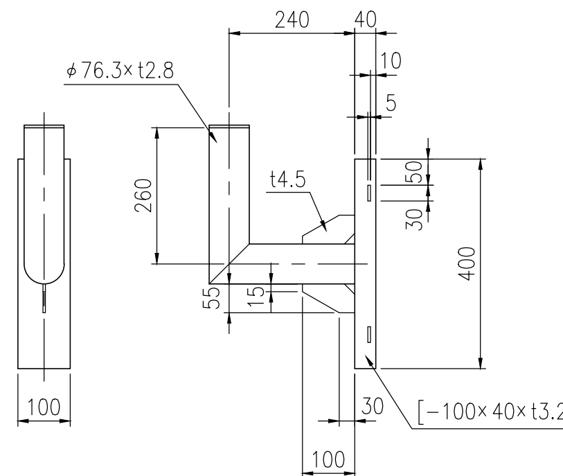
⑧ 電柱取付金具詳細図 S=1/10
