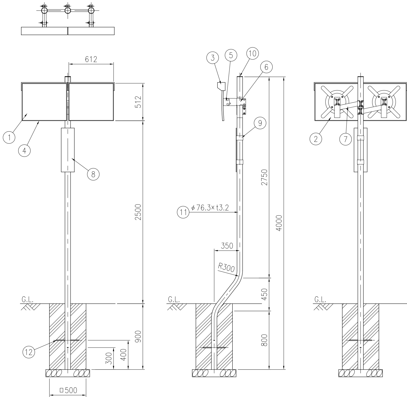
設置図 S=1/25
