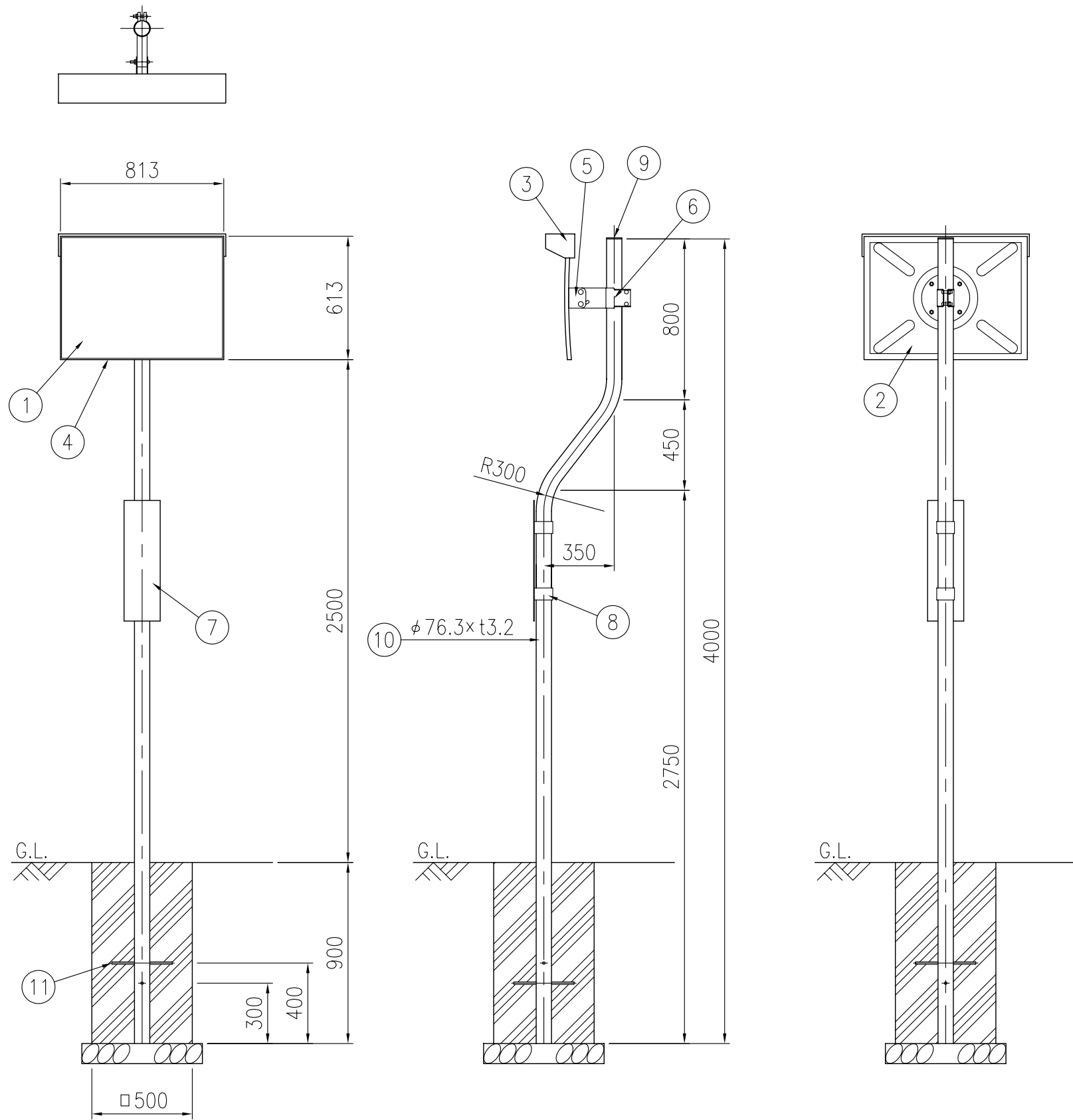
設置図 S=1/25
