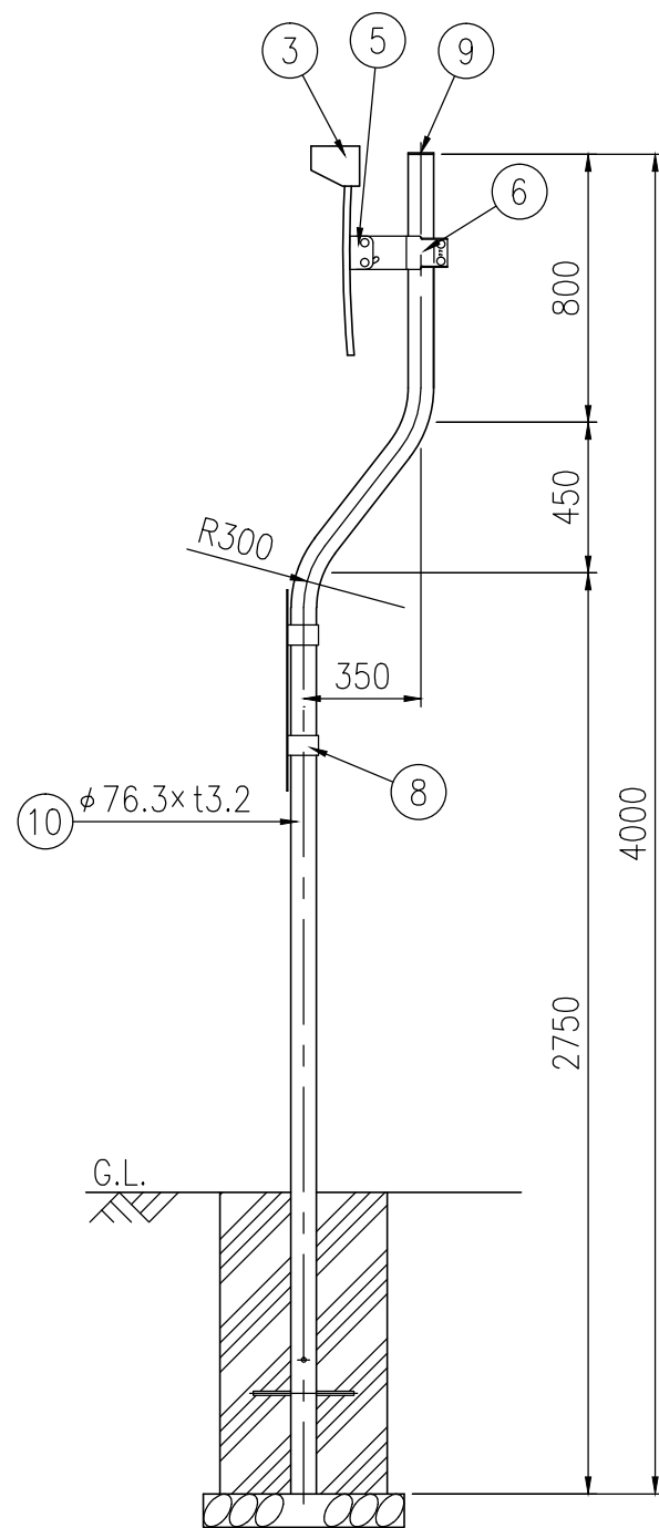
設置図 S=1/25
