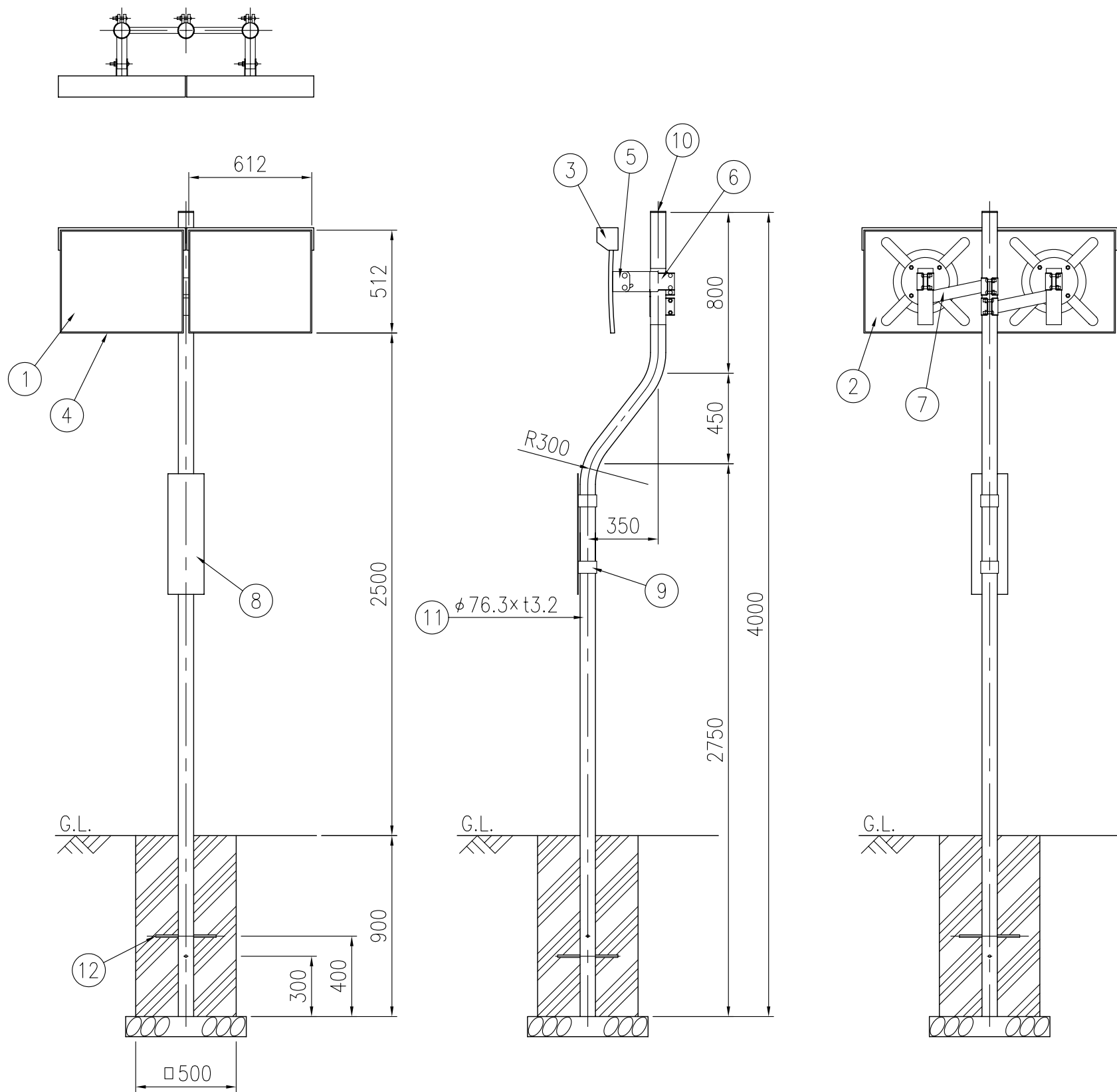
設置図 S=1/25
