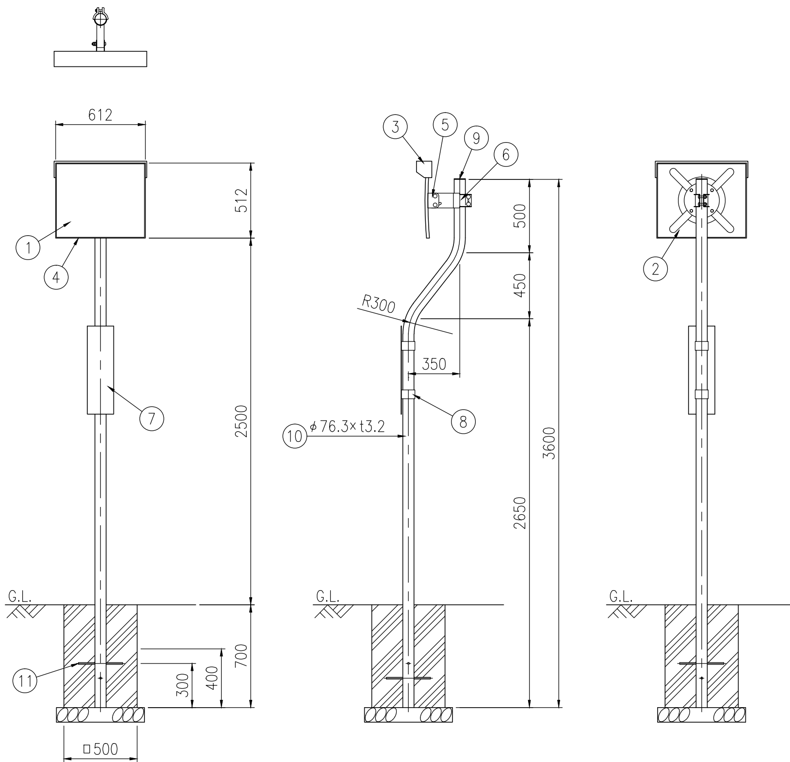
設置図 S=1/25
