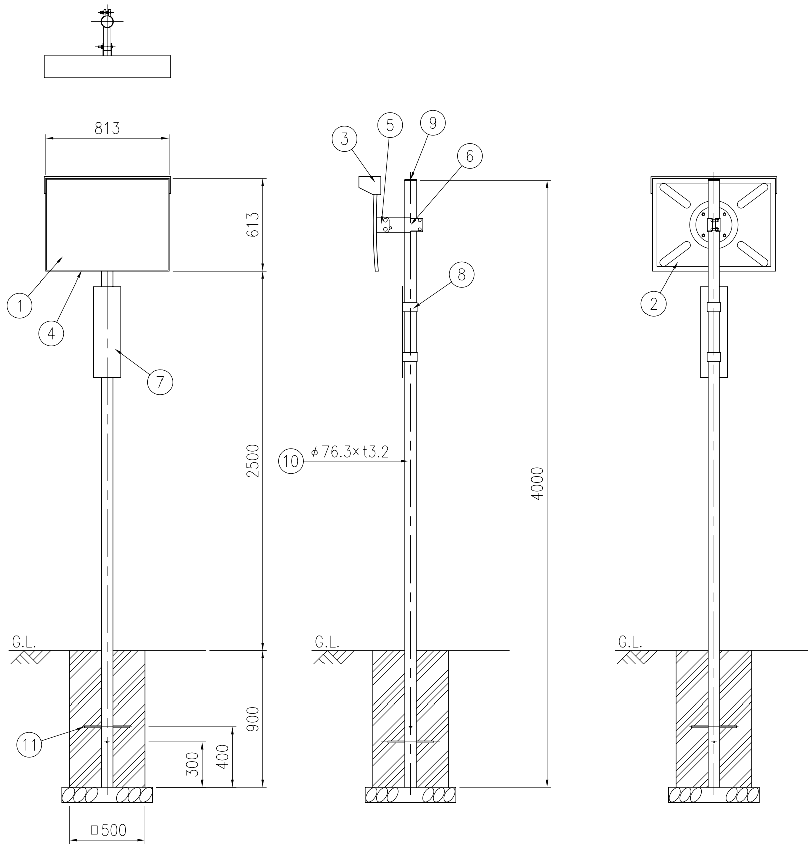
設置図 S=1/25
