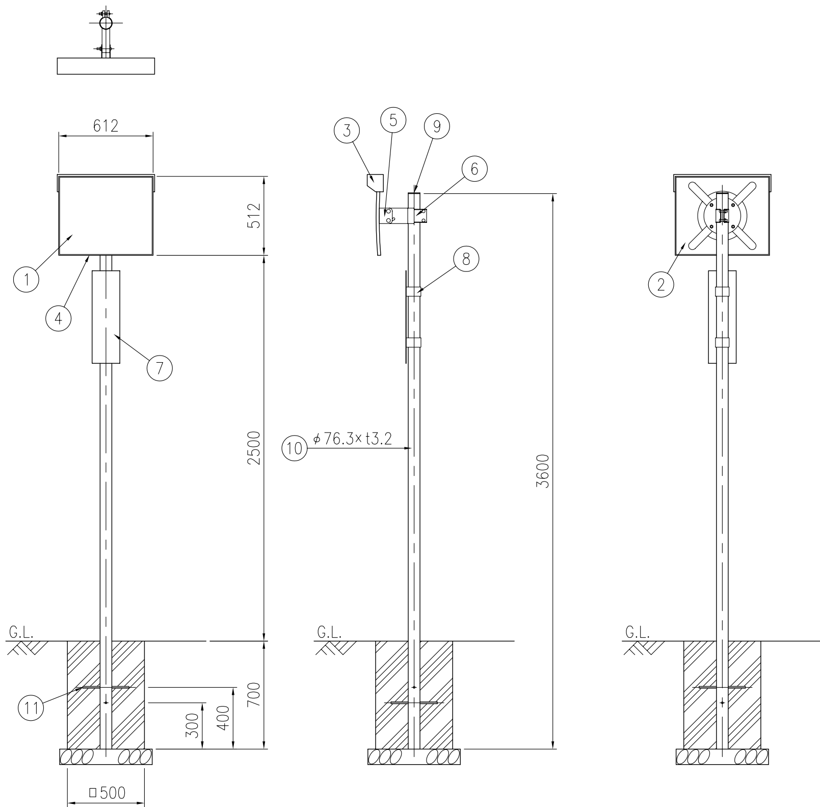
設置図 S=1/25
