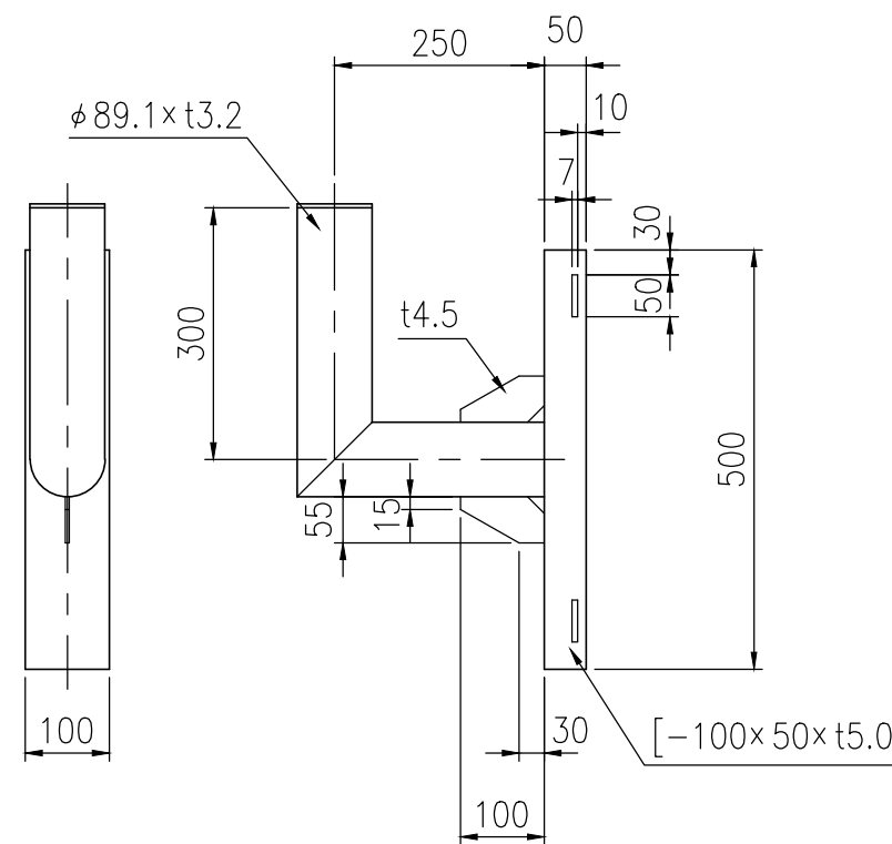
⑧ 電柱取付金具詳細図 S=1/10
