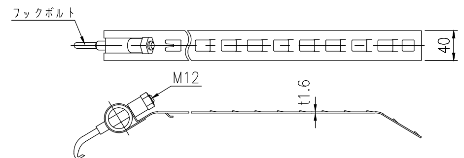
⑩ 取付バンド詳細図 S=1/5
