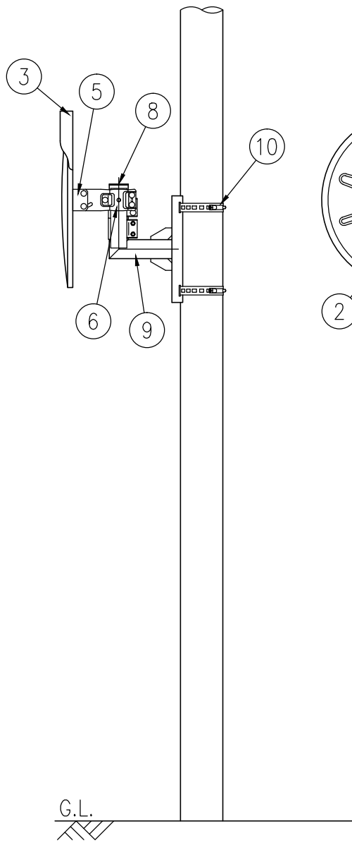
設置図 S=1/25
