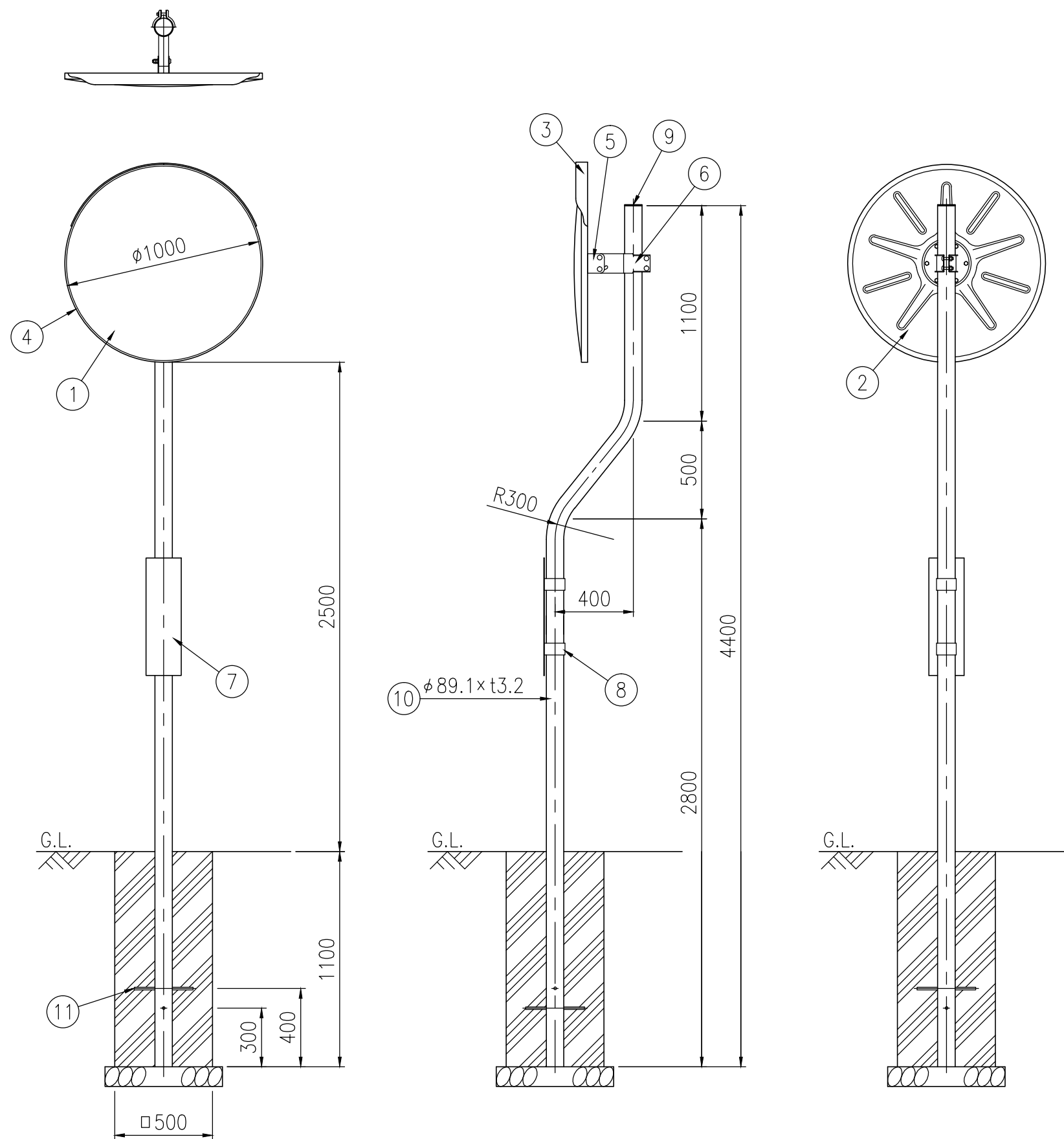
設置図 S=1/25
