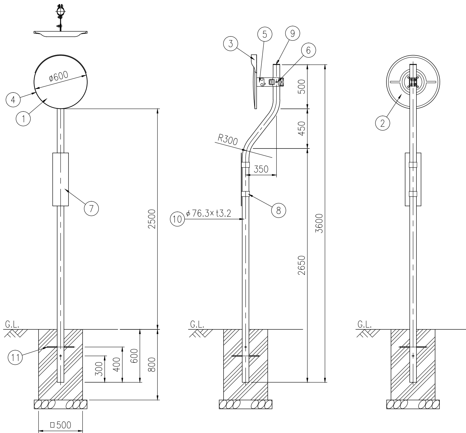
設置図 S=1/25
