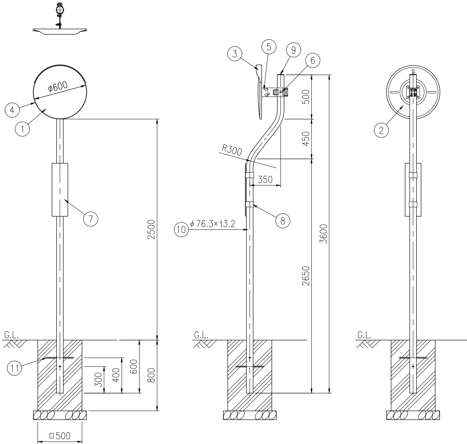
設置図 S=1/25
