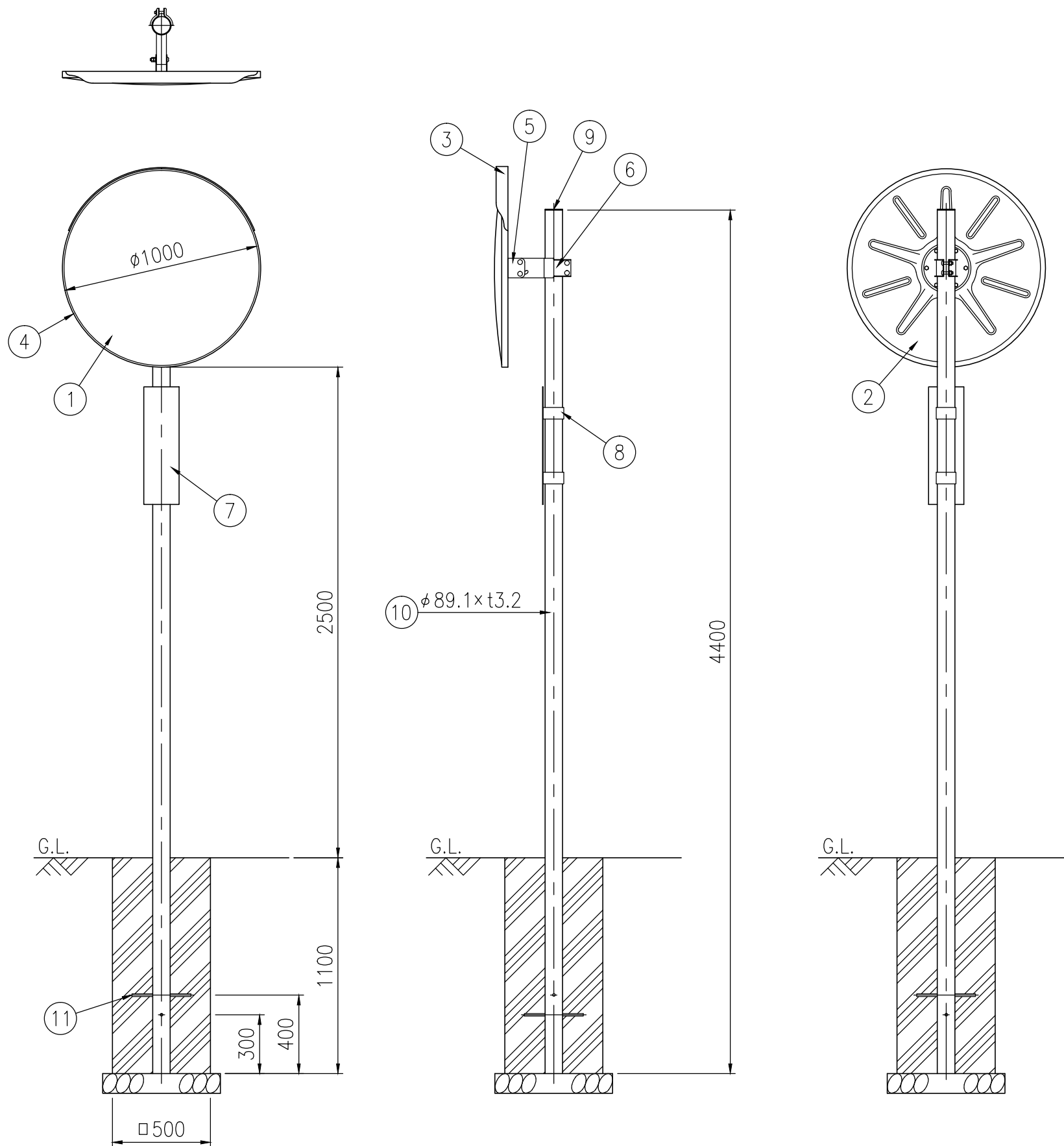
設置図 S=1/25
